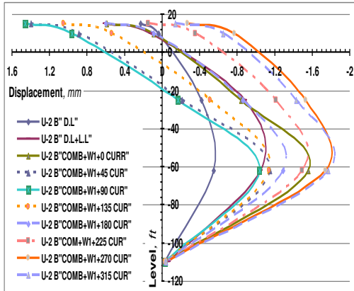
(d) U 2 for Leg B
