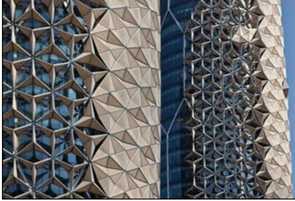
شكل ٦: يوضح استجابة وحدات لتظليل بواجهات مباني أبراج البحر لحركة الشمس فعند سقوط أشعة الشمس عليها تغلق لتحجب أشعة الشمس المباشرة، وعند عدم تعرضها لأشعة الشمس المباشرة فإنها تنطوي لتسمح بدخول الضوء الخارجي الى داخل فراغات المبنى [١٧].
