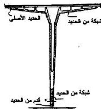
الهيكل الإنشائي للعمود المشرومي في صالة المبنى الإداري [٤١]
